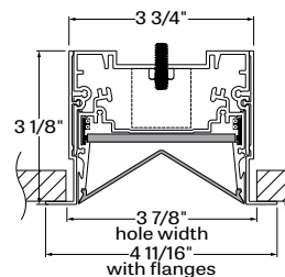
SHL3R-VLO - Drywall trim
