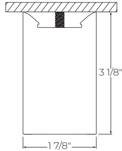
DRC - Drywall ceiling
