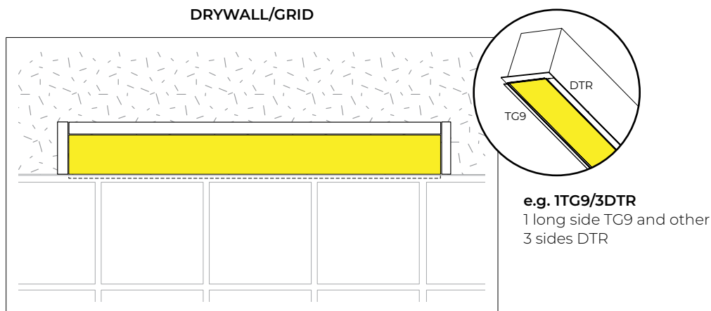
DRYWALL/GRID
